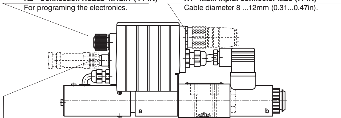
K3 - Conektor M12x1 (5PIN)
